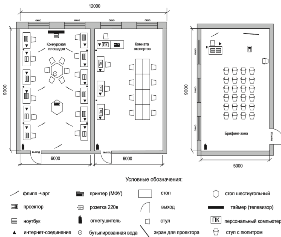
План застройки площадки чемпионата WorldSkills Russia 2020 Алтайского края по компетенции R9 «Туризм»
